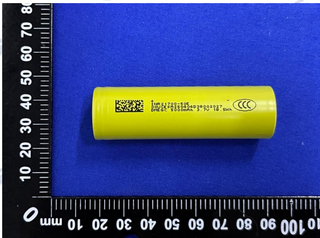
Photo 3 内部电芯 Internal Cell
